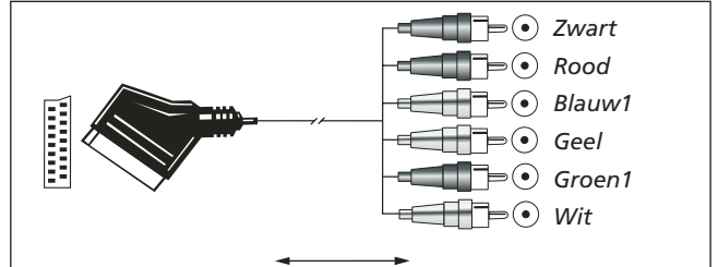
Afbeelding 2: scart/cinch adapter voor opnemen en weergeven; richting: scart ↔ cinch
