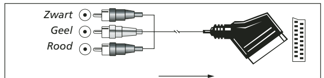
Afbeelding 3: cinchscart adapter voor weergave; richting: cinch → scart
